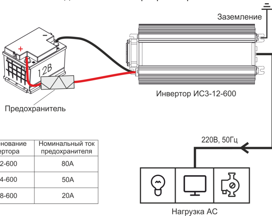
Схема подключения ИС3-24-600.
